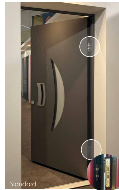
PIÈCES ANTI-DÉGONDAGE pour empêcher le soulèvement de l'ouvrant lors d'une tentative d'effraction
