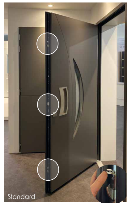
SERRURE MULTIPPOINT Automatique avec 5 points de fermetures : 2 crochets, 2 pènes ronds et un pêne dormant
