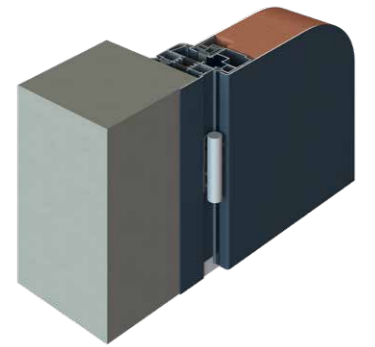
POSE EN BORDS TABLEAU Dormant étroit sans aile + plat de finition
